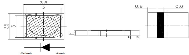
外形图和尺寸
