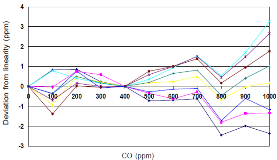
图4 1000ppm线性度
