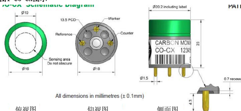
图1 CO-CX图示
